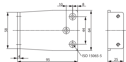
Montážní plech – lomenné ramínko A154
